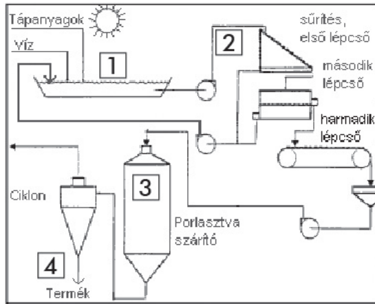
5. ábra: A Spirulina-előállítás folyamata nagyüzemi körülmények között (1. tenyésztés, 2. betakarítás, 3. szárítás, 4. csomagolás)
