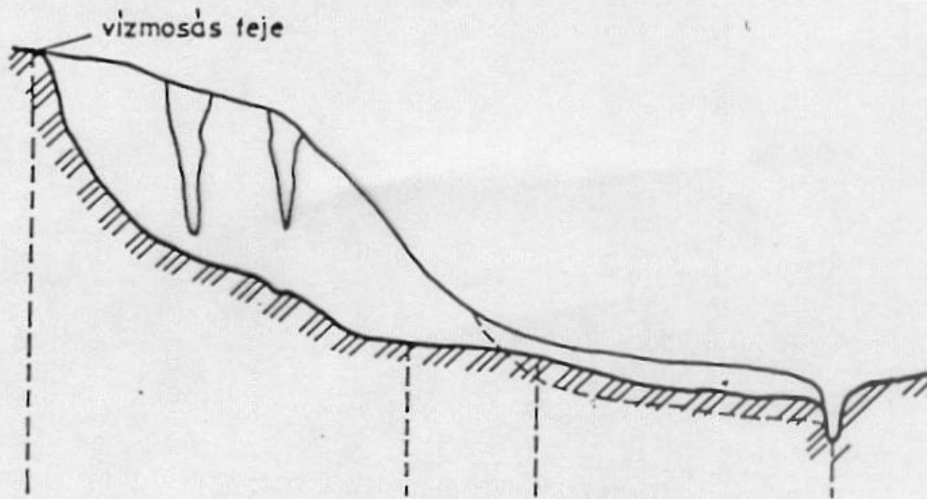
I–3. ábra. Vízmosás helyszínrajza és hossz-szelvénye
